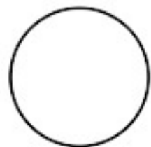
Unknot
